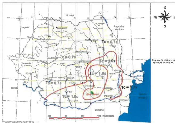
Fig. 3 - Zonarea teritoriului Romaniei in termeni de perioada de control (colț), T_c a spectrului de raspuns
