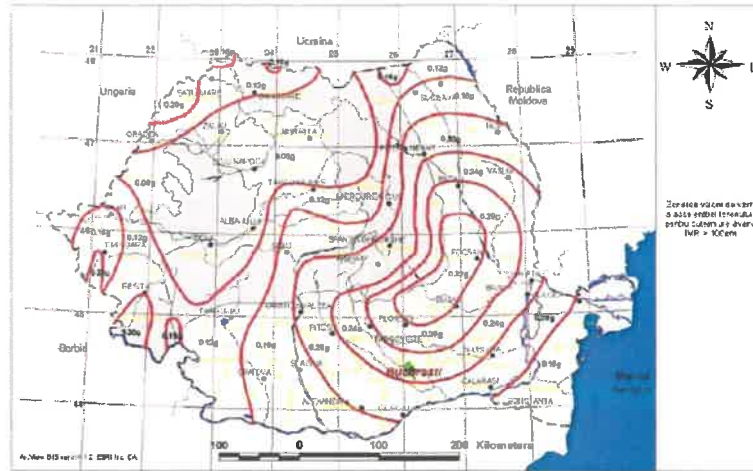
Fig. 2 - Zonarea teritoriului României în termeni de valori de vârf ale accelerației terenului pentru proiectare ag pentru cutremure având intervalul mediu de recurența IMR=100 ani
