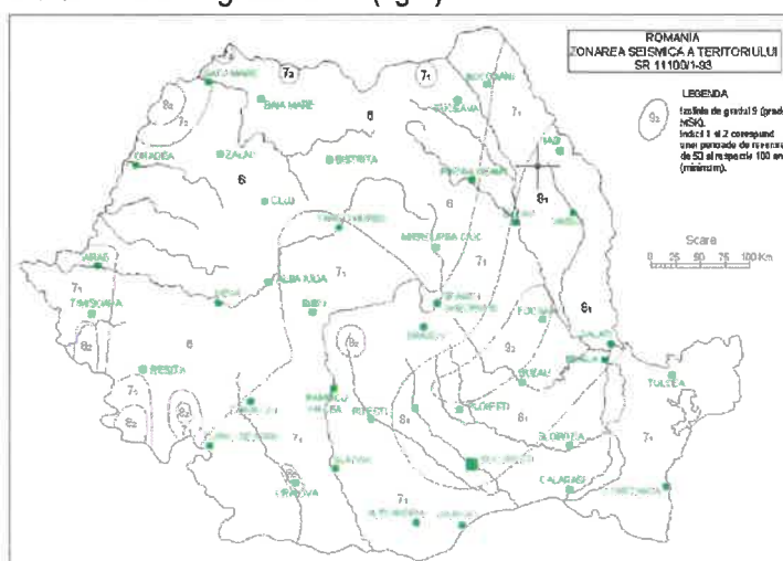
Fig. 1 - Zona seismică a teritoriului României
